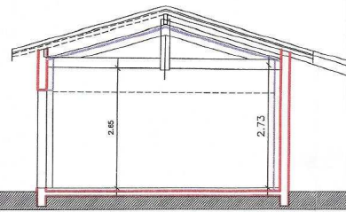
Coupe de Terrain
